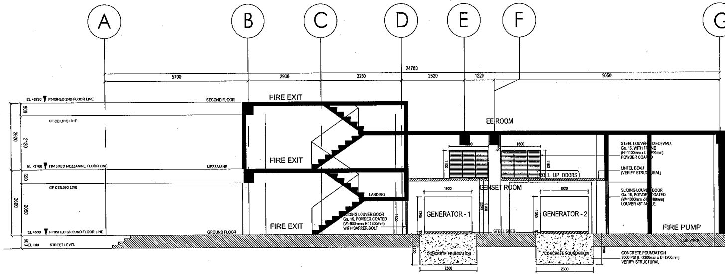
01 SECTION A E1/3 SCALE 1:50 MTS.
