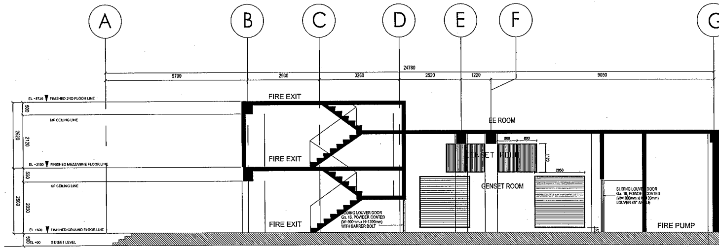
02 SECTION B E1/3 SCALE 1:50 MTS.
